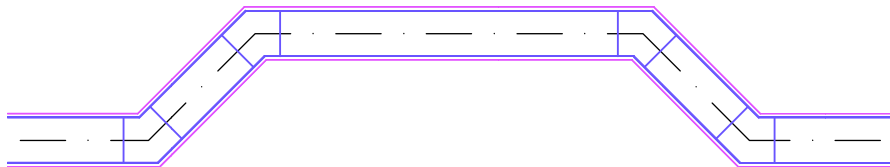
Leitung Gezeichnet mit LEITUNG 3-STRICHE: Schmutzabwasser mit 13mm Isolation
