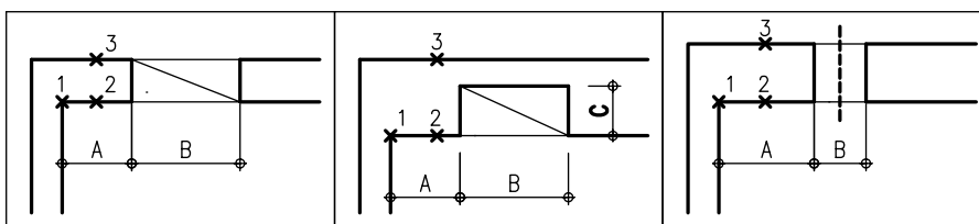
Wanddurchbruch
